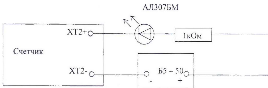
Рисунок 1 – Схема подключения светодиодного индикатора к импульсному выходу при измерении активной энергии
