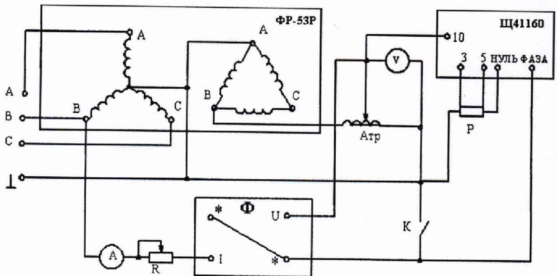
Рисунок 1 – Схема определения основной относительной погрешности измерений силы переменного тока
