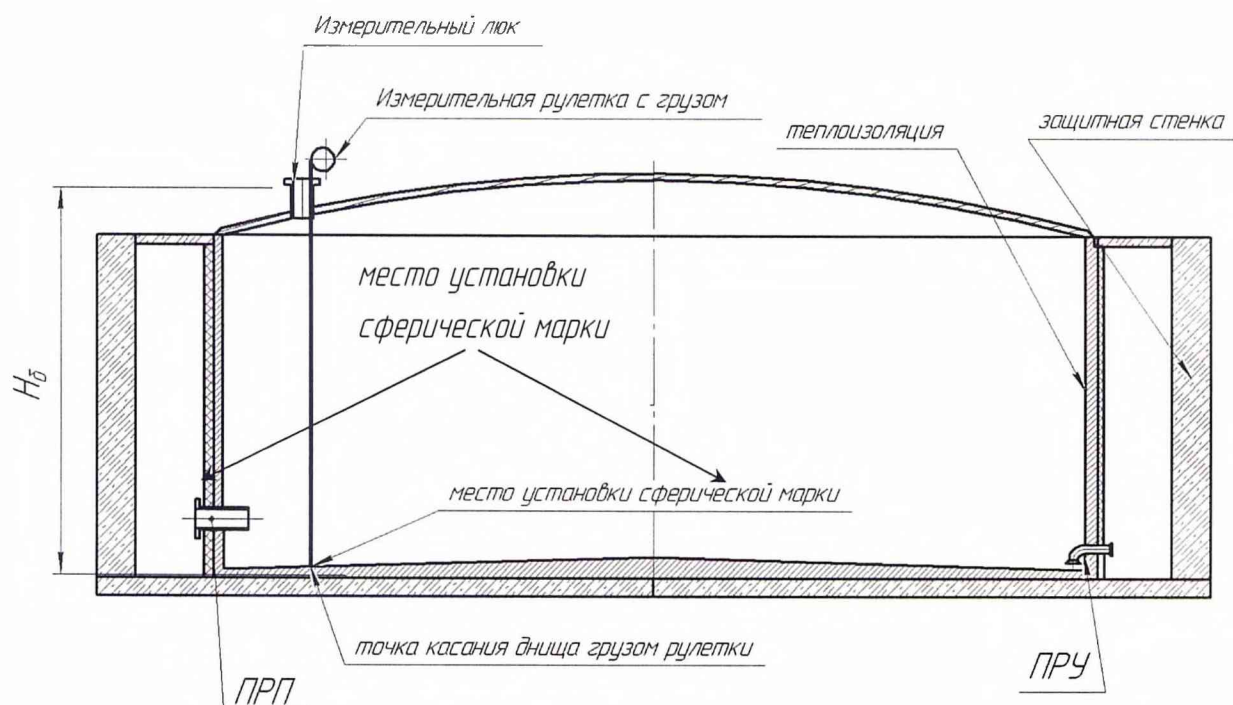
Рисунок А.1 – Общий вид резервуара и схема измерений базовой высоты резервуара
