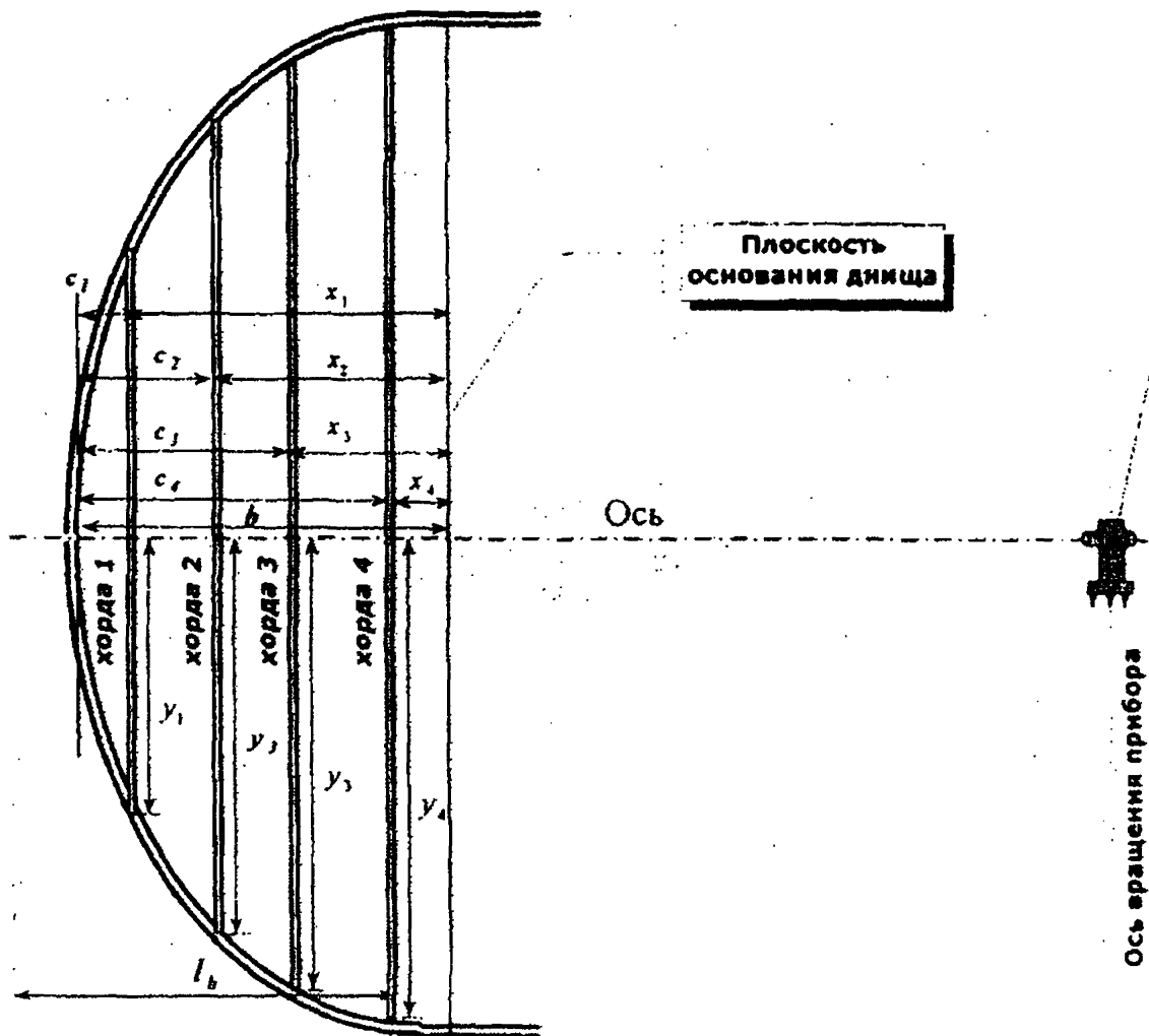
Рисунок А.3 – Определение геометрических параметров днища резервуара
