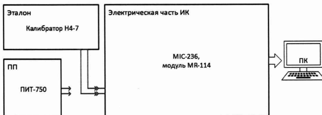
Рисунок 12 – Схема поверки электрической части ИК силы переменного тока
