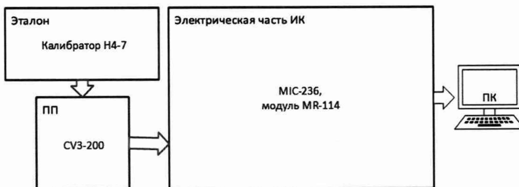
Рисунок 11 – Схема поверки ИК напряжения переменного тока генератора комплектным способом
