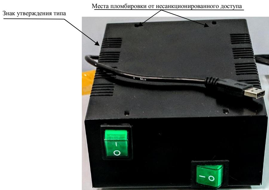
Рисунок 2 – Схема пломбировки от несанкционированного доступа и место размещения знака утверждения типа
