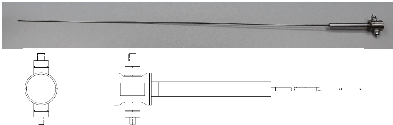
Рисунок 1 - Общий вид преобразователей термоэлектрических 111Т0539Р
