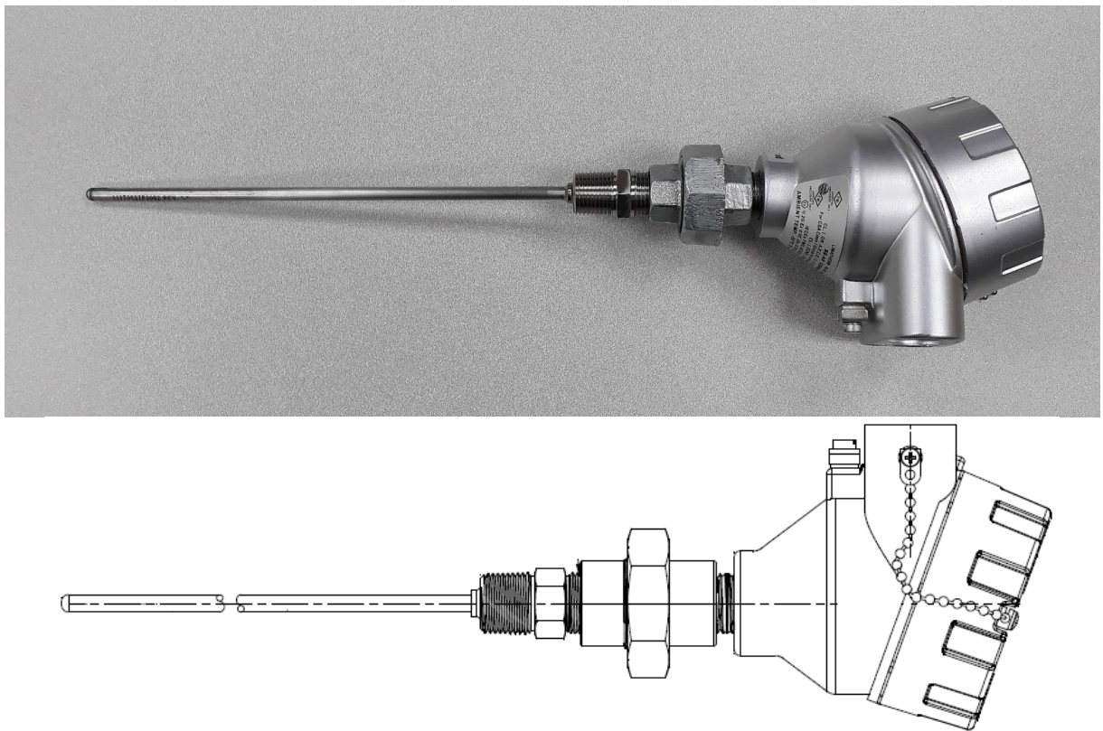
Рисунок 1 - Общий вид преобразователей термоэлектрических модели 111Т0537Р0002
