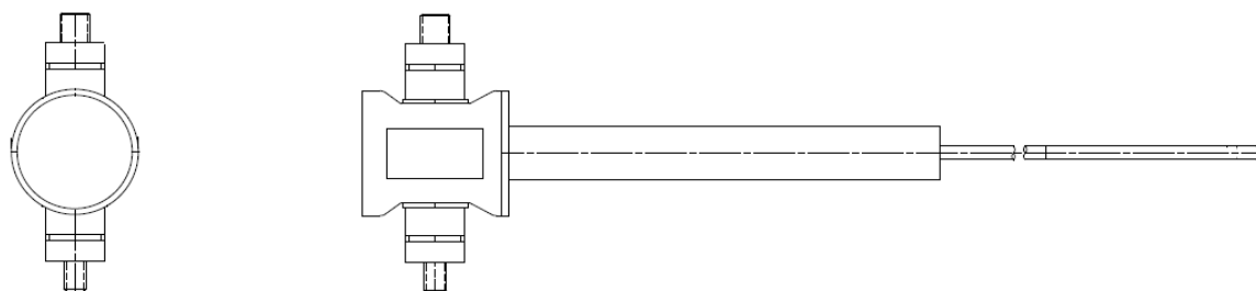
Рисунок 1 - Общий вид преобразователей термоэлектрических модели 111Т0539Р0009
