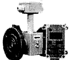
Расходомеры РСЦ
