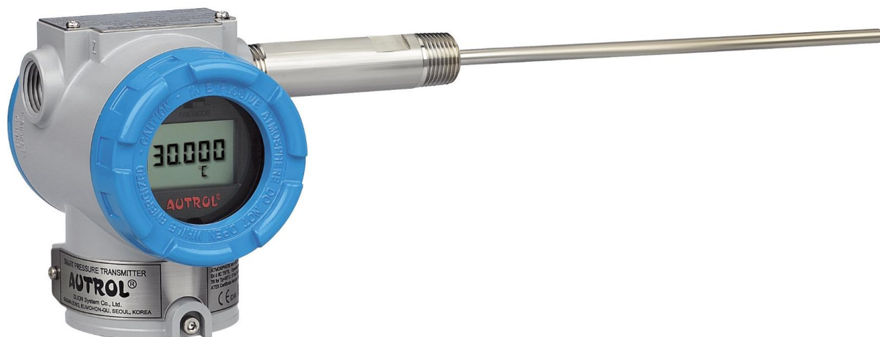
Рисунок 1 - Общий вид датчиков температуры AUTROL модели АТТ2100
