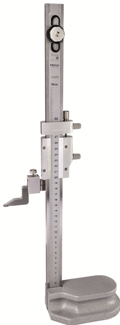
Рисунок 2 – Общий вид штангенрейсмасов серии 514
