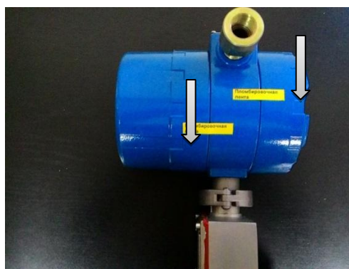
Рисунок 2 - Схема пломбировки от несанкционированного доступа расходомеров Румасс
