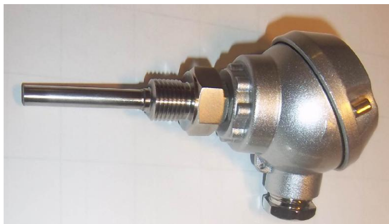
Рисунок 2 – Общий вид термопреобразователей сопротивления платиновых серии 2 модели 2ххJ модификации 211J
