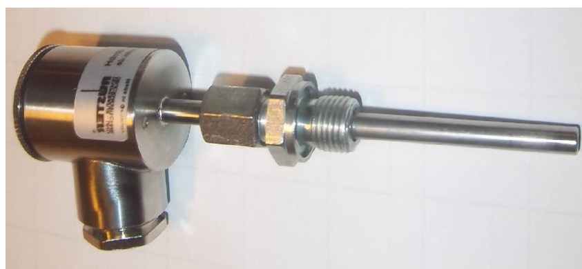
Рисунок 4 – Общий вид термопреобразователей сопротивления платиновых серии 2 модели 2ххBR модификации 212BR30
