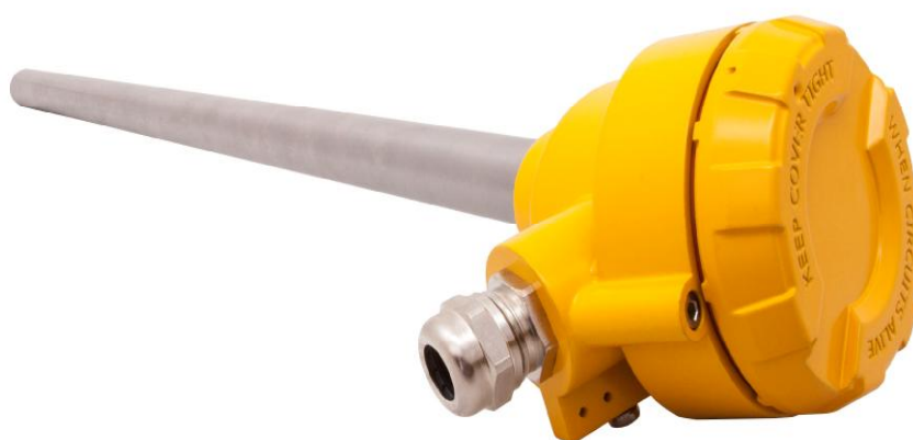
Рисунок 19 - Внешний вид ТП СТУ с защитным корпусом из нержавеющей стали
