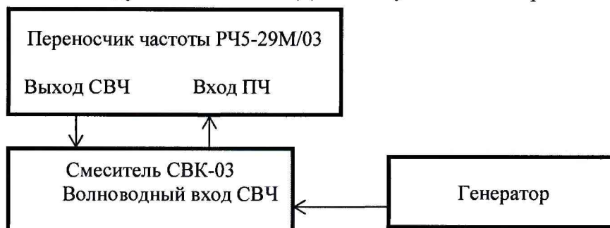
Рисунок 2 - Схема подключений
