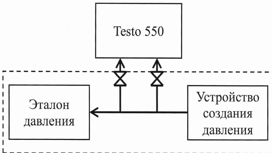
Рисунок А.1 -Схема соединения для определения погрешности измерений избыточного давления без разделительной камеры
