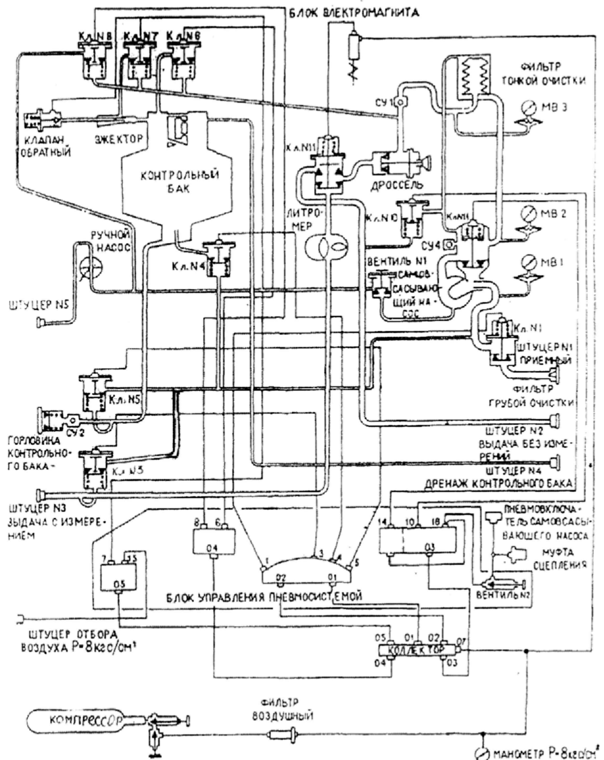
Рисунок А.1 – принципиальная гидропневматическая схема КТР «Зонд».
