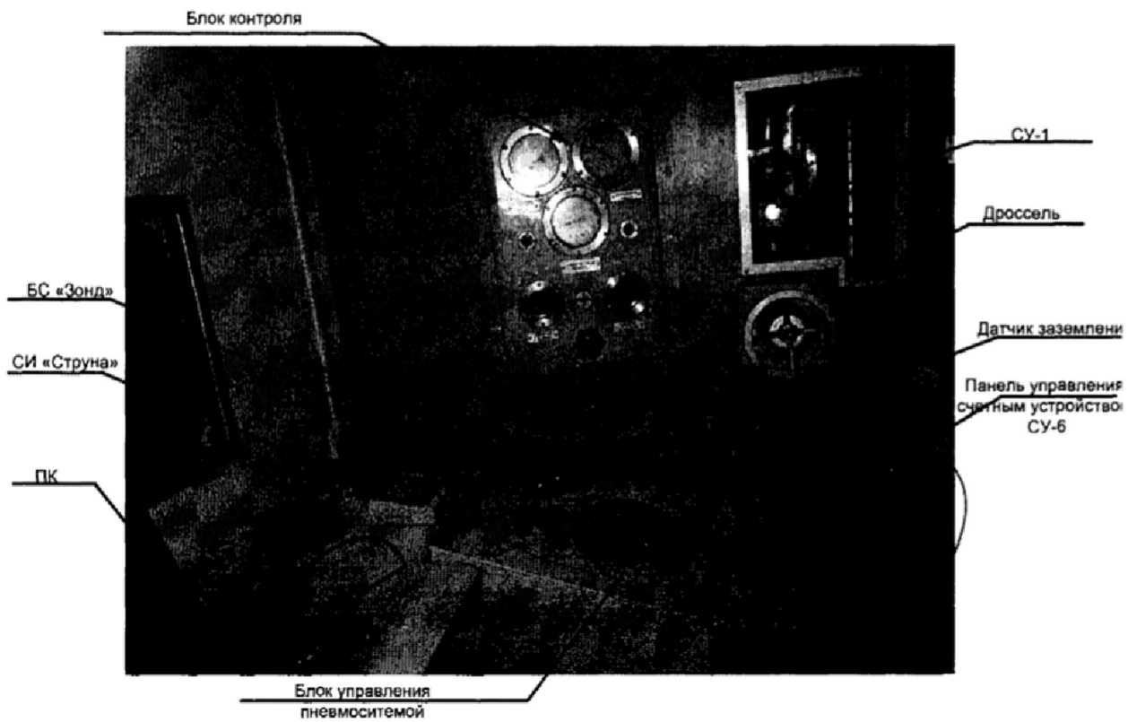
Рисунок А.4 – операторская КТР «Зонд».
