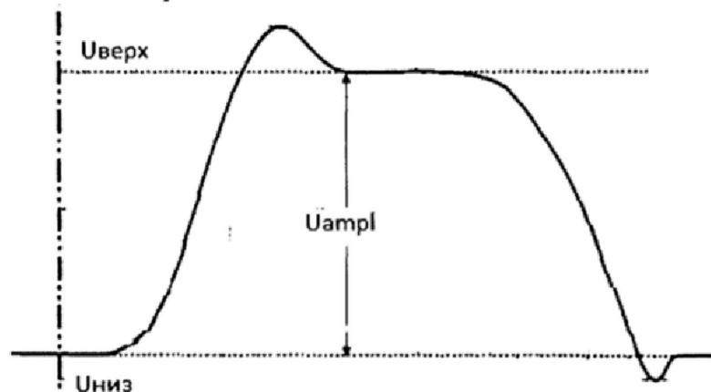
Рисунок 2 - Измерение разности между верхним и нижнем уровнем сигнала (U ampl )
