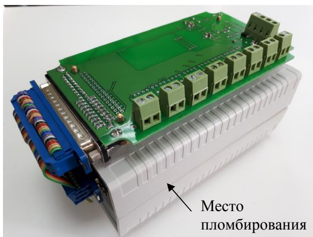
Рисунок 6 - Общий вид приборов Flash-Recorder-3 M4
