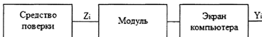
Рисунок 1 - Схема подключений при определении погрешностей ИК, реализующих линейное аналого-цифровое преобразование сигналов силы или напряжения постоянного электрического тока, электрического сопротивления, частоты следования импульсов
