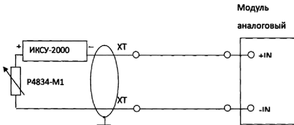
Рисунок Б.2 – Подключение калибратора ИКСУ-2000 и магазина сопротивлений Р4834-М1 к линиям связи со шкафом СКУиР в режиме воспроизведения силы постоянного тока (4 ... 20 мА) (активный режим)
