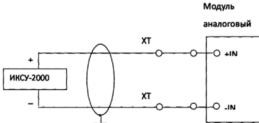
Рисунок Б.1 – Подключение калибратора ИКСУ-2000 к линиям связи со шкафом СКУиР в режиме воспроизведения сопротивления и напряжения постоянного тока
