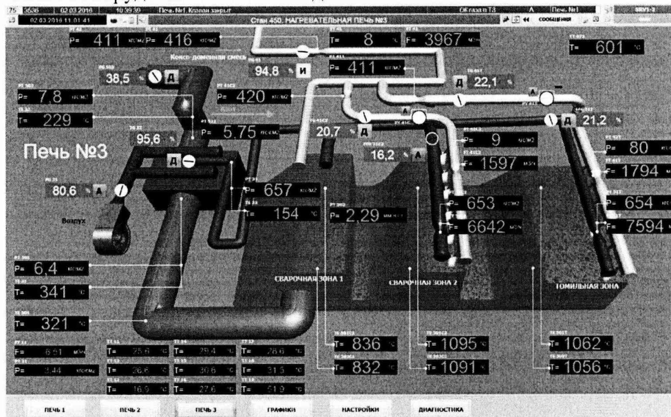
Рисунок 1 – Отображение значений технологических параметров на экранной форме «Стан 450. Нагревательная печь «№ 3»
