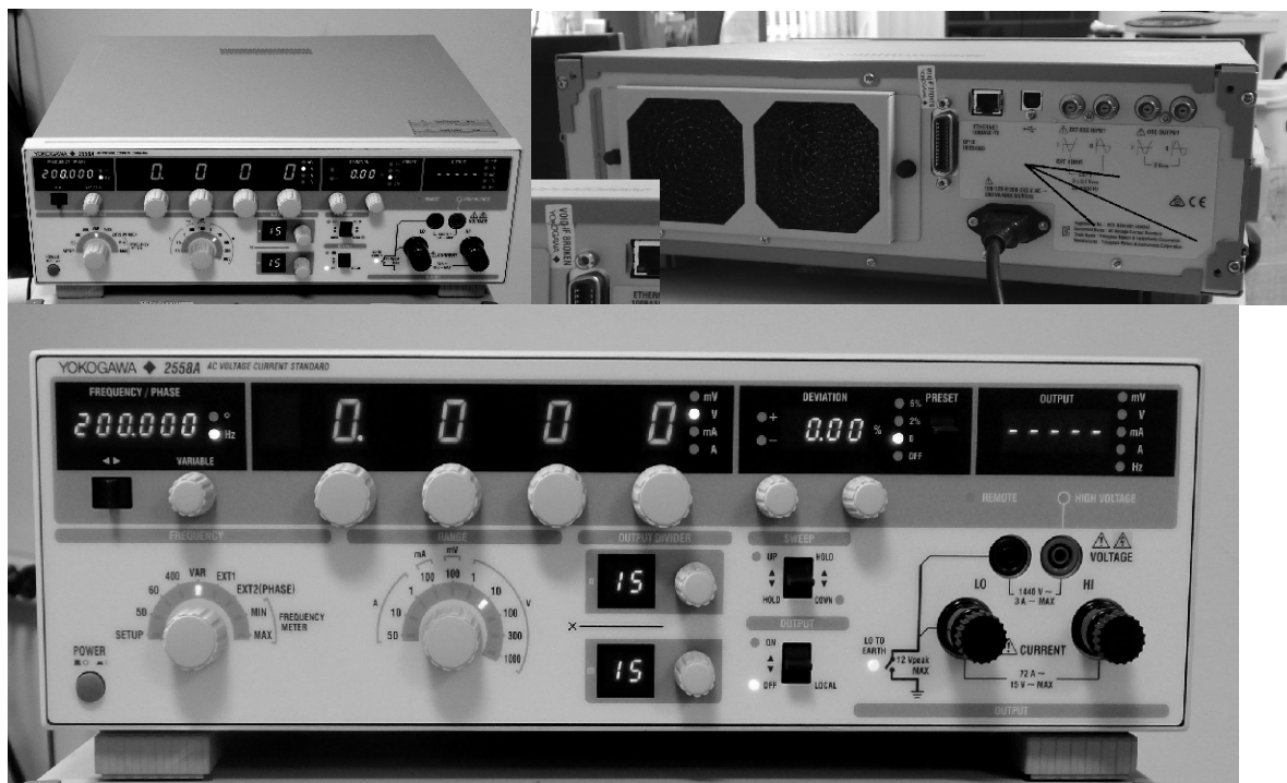
Рисунок 1 - Внешний вид источников напряжения и силы переменного тока эталонных 2558А
