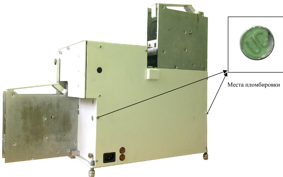
Рисунок 2 - Места пломбировки корпуса дефектоскопа
