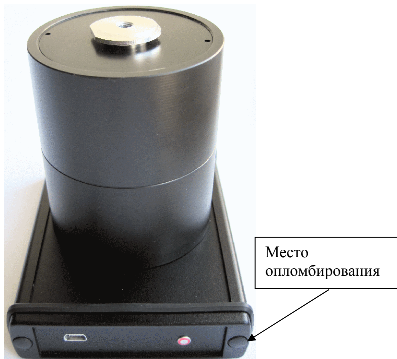
Рисунок 1- Внешний вид устройств воспроизведения вибрации КВ-160
