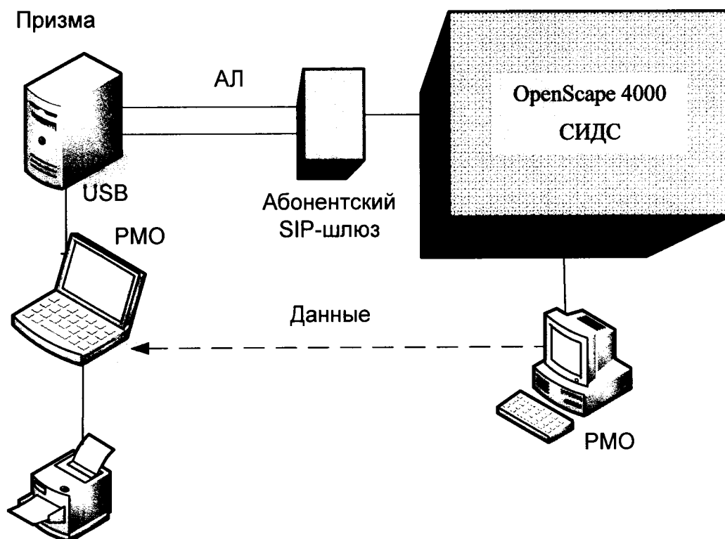
Рисунок 2 - Схема поверки СИДС через абонентский SIP-шлюз
