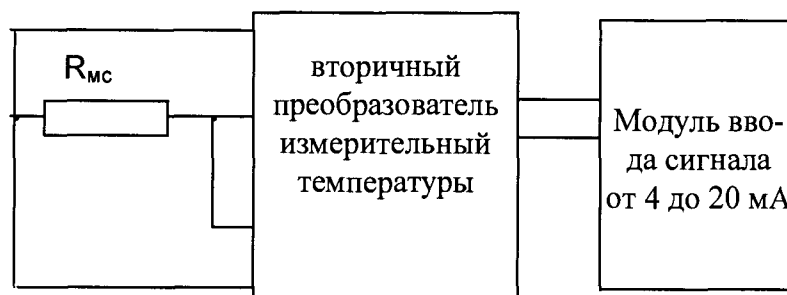
R_{мс} – магазин сопротивлений
