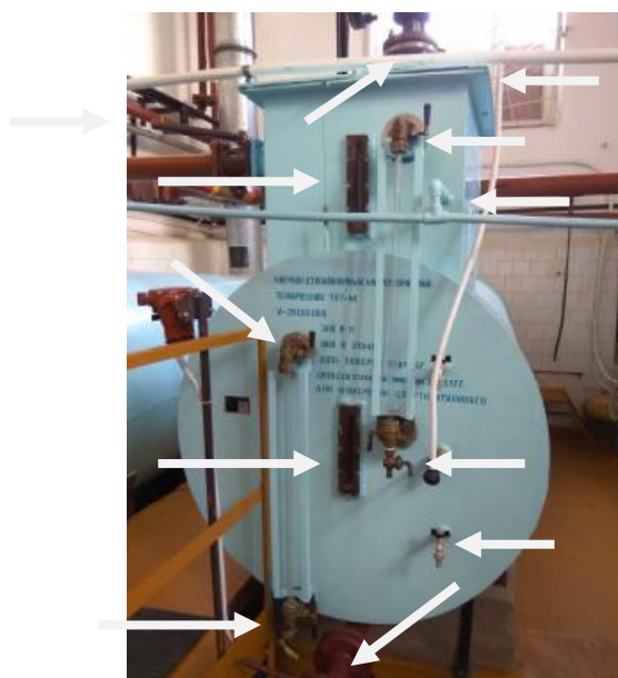
Рисунок 1 - Общий вид и места пломбирования мерника
