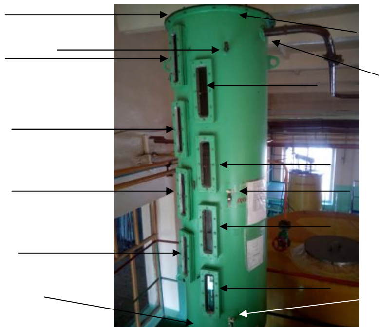
Рисунок 1 - Общий вид и места пломбирования мерника
