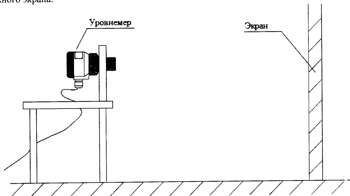
Рисунок 1 – Положение уровнемера при поверке
