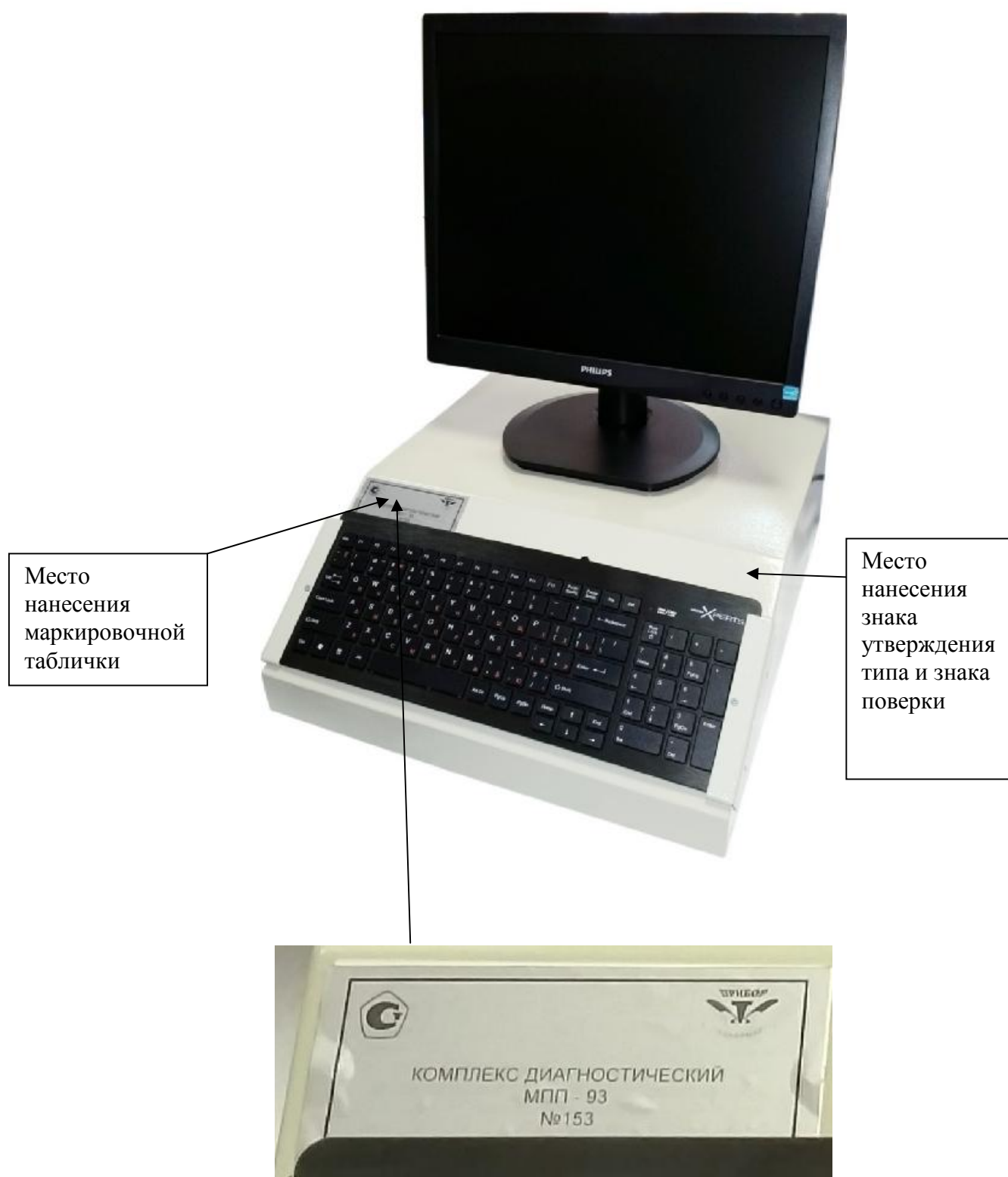
Рисунок 1- Внешний вид информационно-измерительного блока (ИИБ) совместно с монитором и маркировочной табличкой
