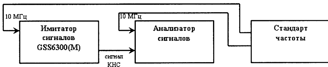
Рисунок 2 – Схема измерений для определения уровня гармонических составляющих
