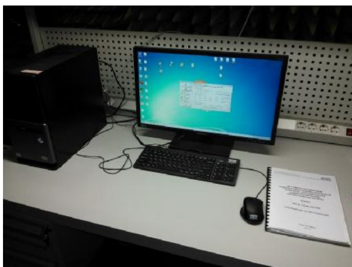
Рисунок 5 – Внешний вид рабочего места оператора с ПЭВМ, предназначенной для управления работой комплекса и обработки результатов измерений
