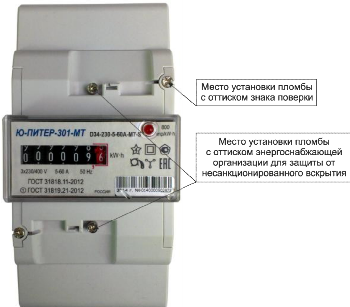
Рисунок 6 – Общий вид счетчика в корпусе модификации D34
