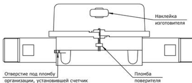
Рисунок 2 – Схема пломбировки счетчиков
