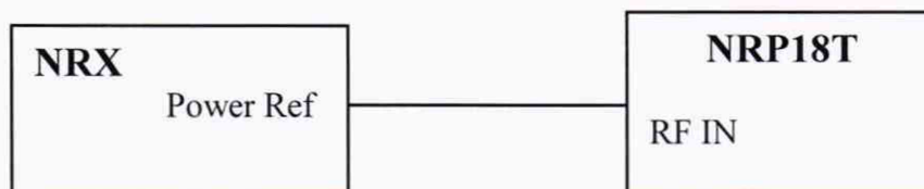
Рисунок 2 - Схема определения основной относительной погрешности установки уровня выходного сигнала NRX
