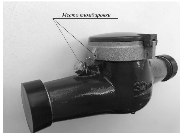
Рисунок 3 - Место пломбировки счетчиков СВ-25В, СВ-25С, СВ-32В, СВ-32С, СВ-40В, СВ-40С, СВ-50В, СВ-50С
