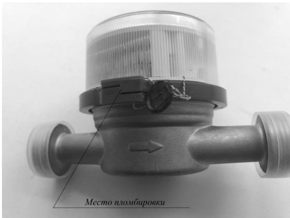
Рисунок 2 - Место пломбировки счетчиков СВ-15В, СВ-15С, СВ-20В, СВ-20С
