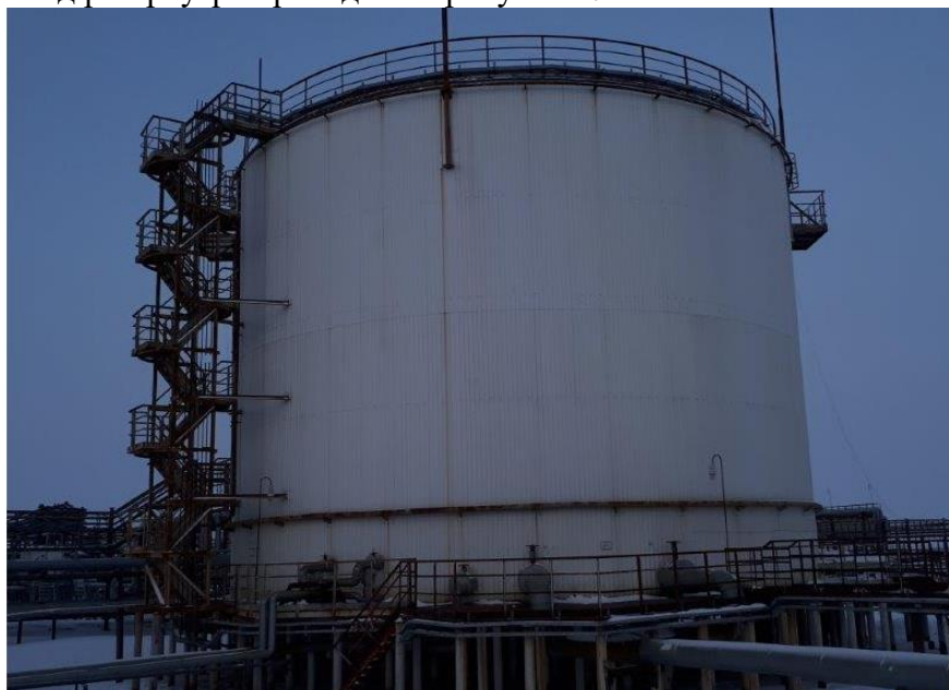
Рисунок 1 – Общий вид резервуара стального вертикального цилиндрического теплоизолированного РВС-5000
