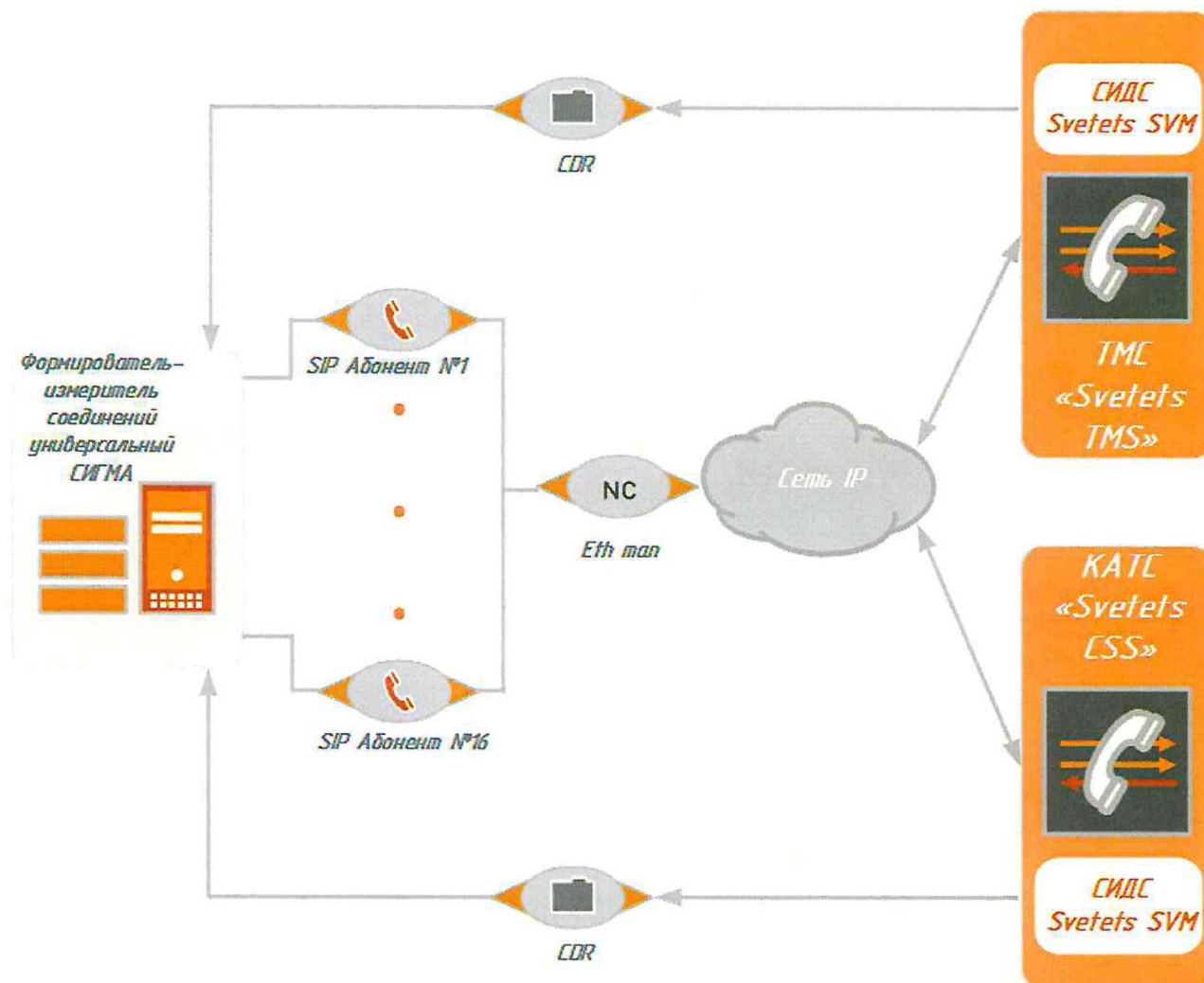
Рисунок 1. Схема поверки
