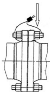
Рисунок 3 – Схема пломбировки от несанкционированного доступа, обозначение места нанесения знака поверки на фланцевые соединения средства измерений массы, объема и плотности жидкости установок
