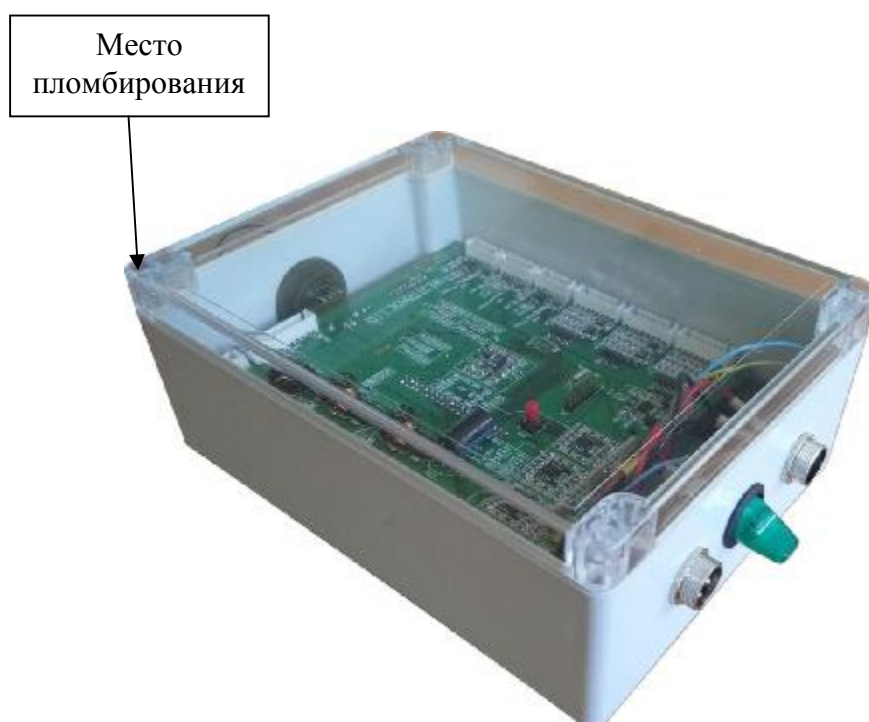
Рисунок 1 - Внешний вид и место пломбирования корпуса от несанкционированного доступа блока приема и передачи сигналов
