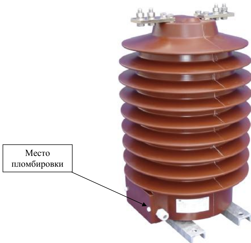
Рисунок 2 – Общий вид трансформаторов тока GIF 12, GIF 24, GIF 40,5
