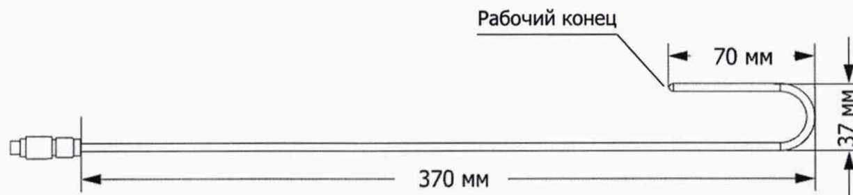
Рисунок Б.1 — Термопреобразователь сопротивления LTA-ДВ
