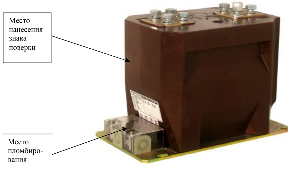
Рисунок 1 – Общий вид трансформаторов тока СТ12
