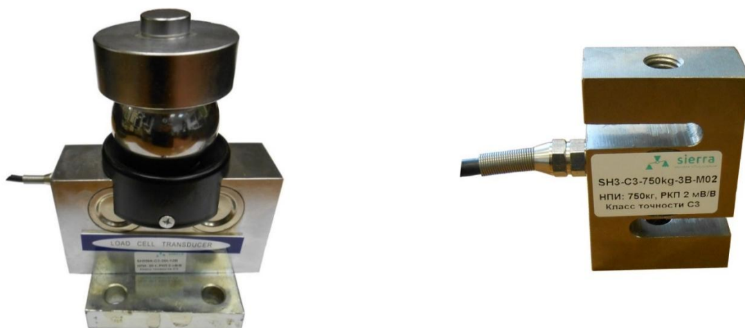
а) семейство Dual shear beam (модификация SHM9) б) семейство S beam (модификация SH3)
