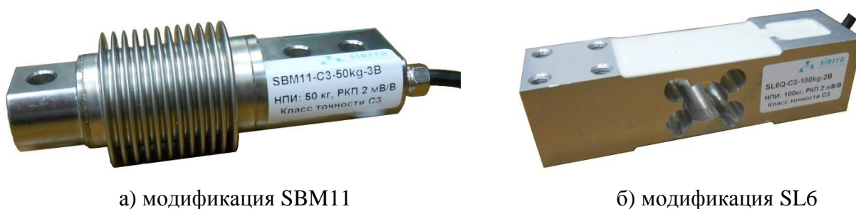
Рисунок 1 – Общий вид датчиков семейства Bend beam
