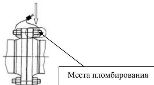
Рисунок 2 – Схема пломбировки от несанкционированного доступа, обозначение места нанесения знаков поверки на фланцевые соединения расходомеров установки поверочной СПРУТ 50М
