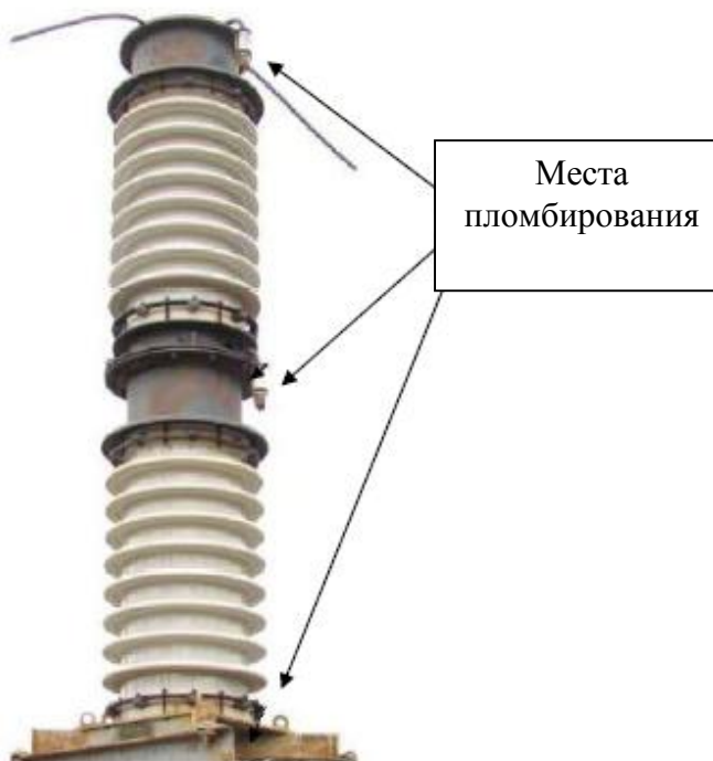
Рисунок 1 – Общий вид трансформаторов напряжения НКФ-220-58ХЛ1 с указанием мест пломбирования
