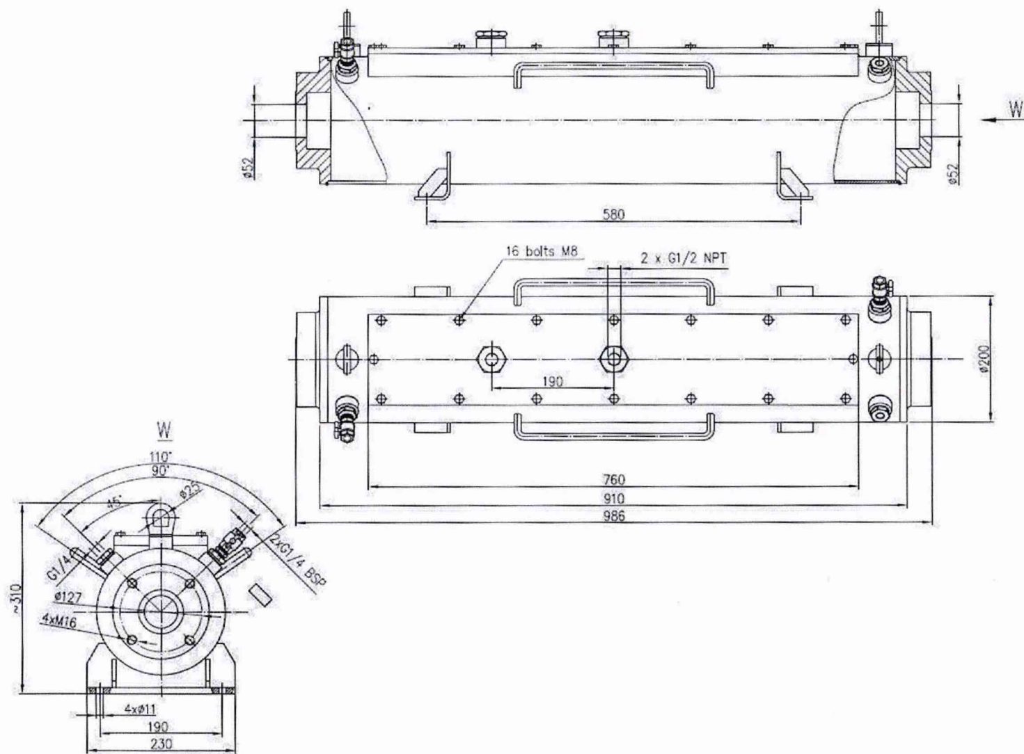
Пример чертежа и габаритных размеров Нулевой камеры.
