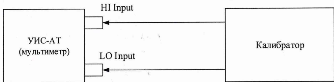
Рисунок 4 – Структурная схема соединения приборов при проверке погрешности измерений напряжения постоянного и переменного тока
