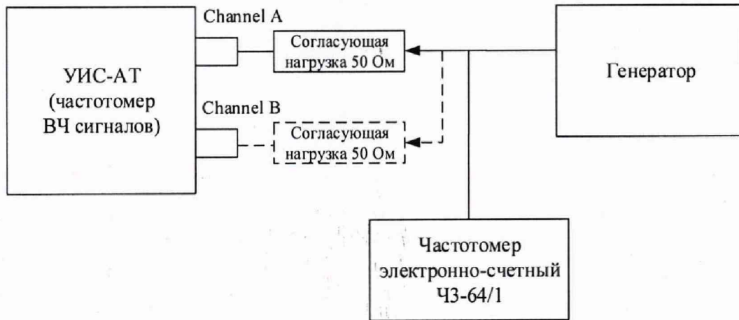
Рисунок 8 – Схема подключения оборудования для проверки частотомера ВЧ сигналов
