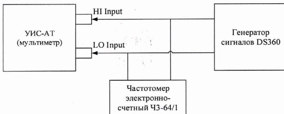
Рисунок 7 – Структурная схема соединения приборов при проверке погрешности измерений частоты
