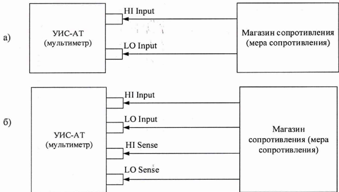
Рисунок 6 – Структурная схема соединения приборов при проверке погрешности измерений сопротивления: а – двухпроводная схема, б – четырёхпроводная схема
