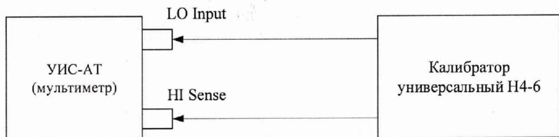
Рисунок 5 – Структурная схема соединения приборов при проверке погрешности измерений силы постоянного и переменного тока
